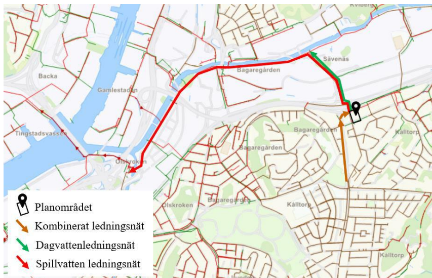
Karta över avrinningsområden och dagvattenförande ledningssystem. Svart fyrkant visar avledningen från planområdet.
