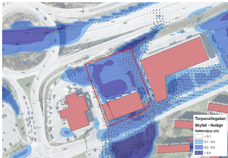
Skysfallssituationen vid planområdet i nuläge. Blå färgen visar vattendjup vid klimatanpassat regn med 100 års återkomsttid.
